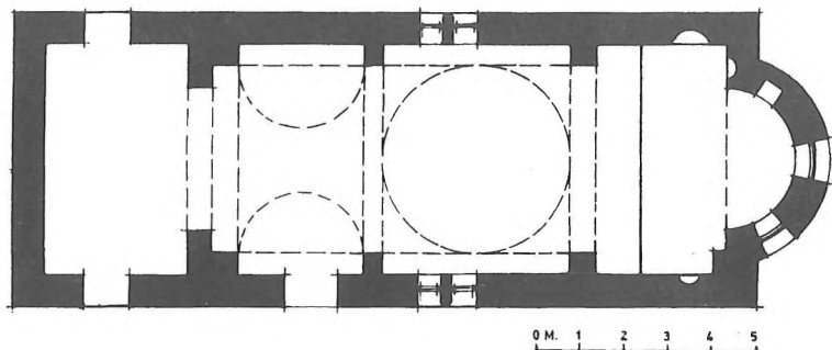
Εἰκ. 27. Ἡ κάτοψις τῆς μονόκλιτου τρουλλαίας βασιλικῆς τῆς Κοιμήσεως.
