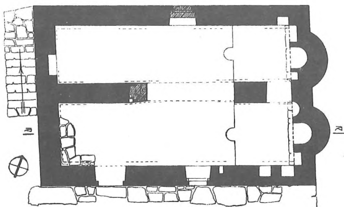
ΚΑΤΟΨΙΣ
