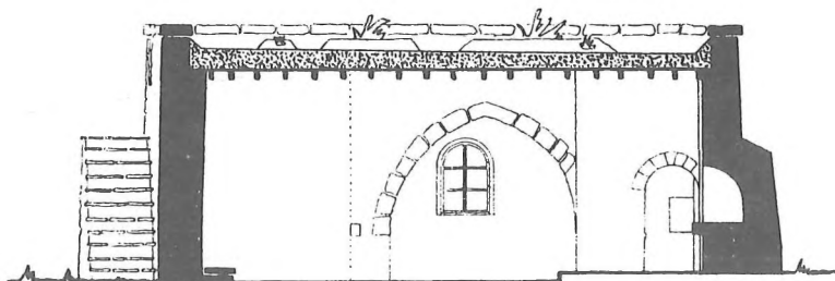
Τομή αβ
