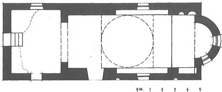
Εἰκ. 33. Ἡ κάτοψις τῆς μονόκλιτου τρολλαίας βασιλικῆς τῶν Ταξιαρχῶν.
