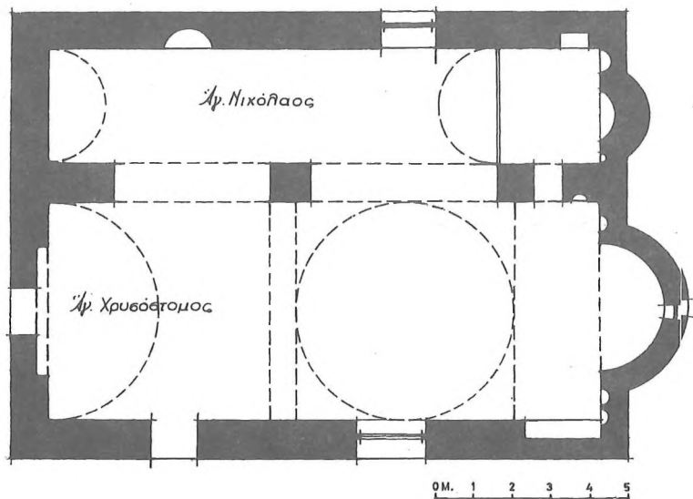
Εἰκ. 22. Ἡ κάτοψις τοῦ δικλιτοῦ ναοῦ τοῦ Χρυσσοστόμου.
