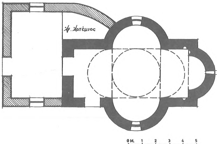
Εἰκ. 18. Ἡ κάτοψις τοῦ ἀπλοῦ τρίκογχου ναοῦ τῆς Εὐαγγελιστρίας.
